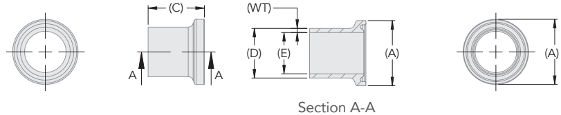
Section A-A
